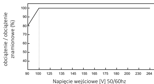
CHARAKTERYSTKA OBCIĄŻALNOŚCI W ZALEŻNOŚCI OD NAPIĘCIA WEJŚCIOWEGO
